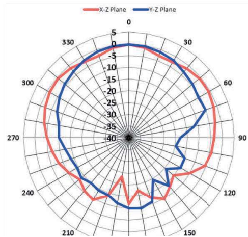
6.5GHz
