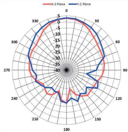
5.5GHz
