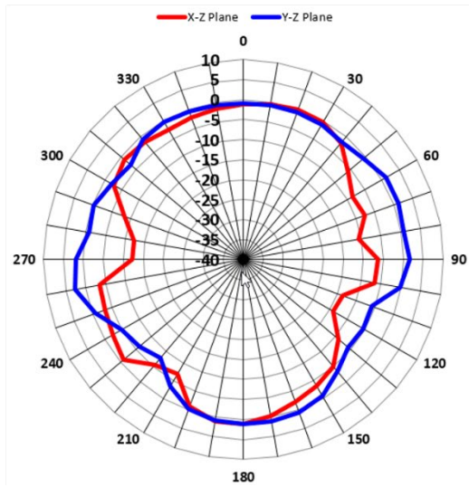
0.6GHz_Horizontal
