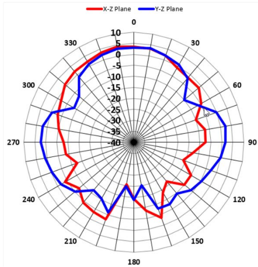
6.5GHz_Horizontal
