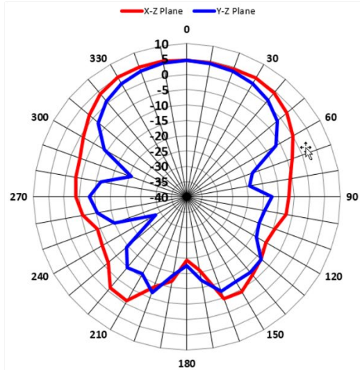
4.5GHz_Horizontal
