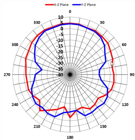
3.5GHz_Horizontal
