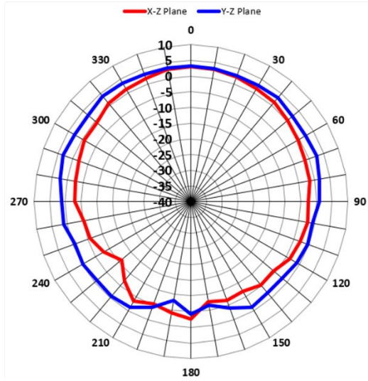
1.8GHz_Horizontal
