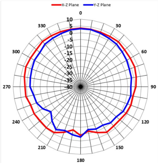
1.8GHz_Vertical
