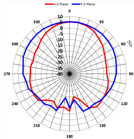
2.4GHz_Horizontal
