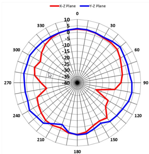
0.9GHz_Horizontal
